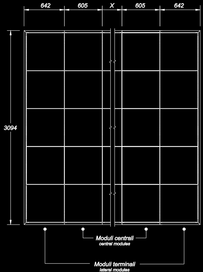
5 moduli/modules (h 3094 mm)
