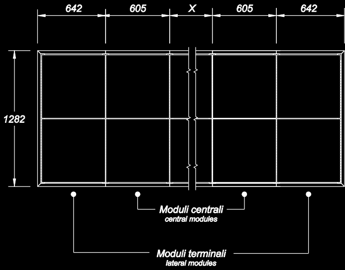
2 moduli/modules (h 1282 mm)
