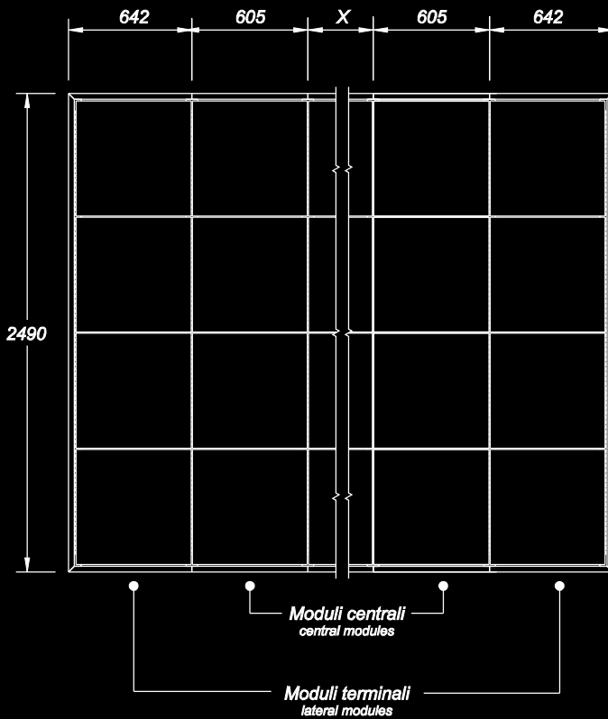
4 moduli/modules (h 2490 mm)
