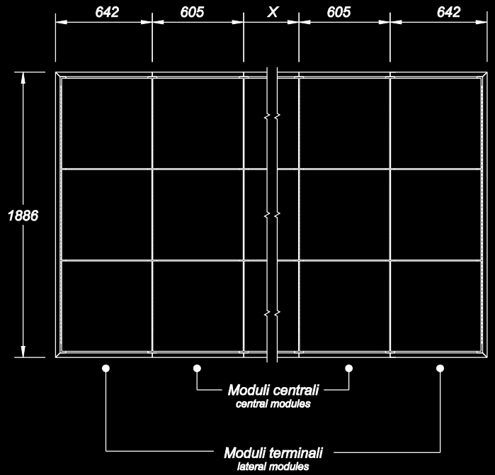
3 moduli/modules (h 1886 mm)
